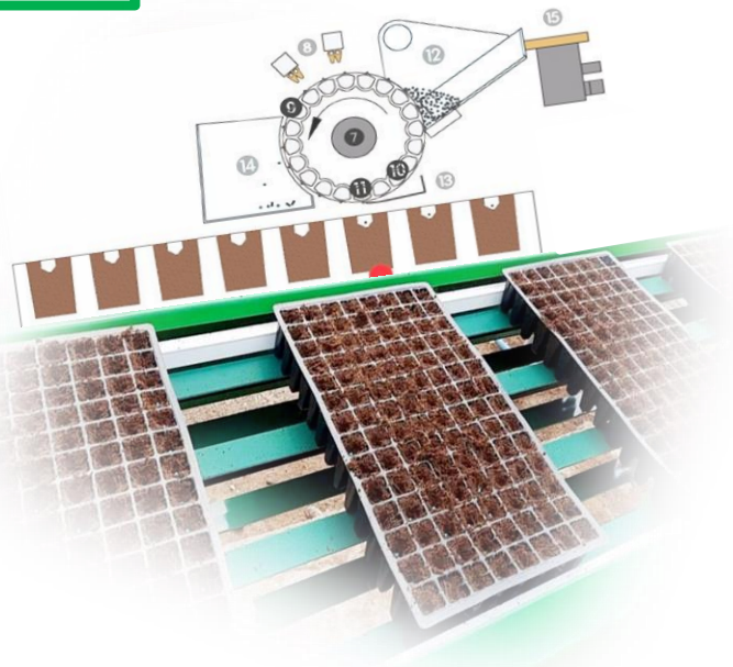
درايم کارنده قسم زارع Seeding drum
